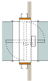
Exempel lättregelvägg
