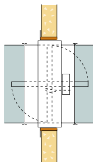
Exempel schaktvägg
