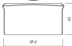
Nippelanslutning
